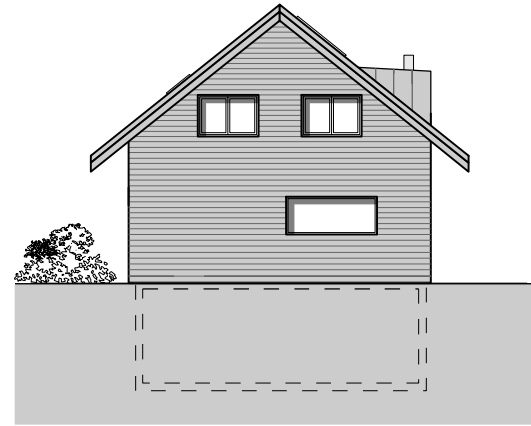
Façade Ouest
