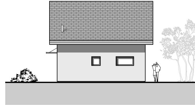
Façade Ouest
