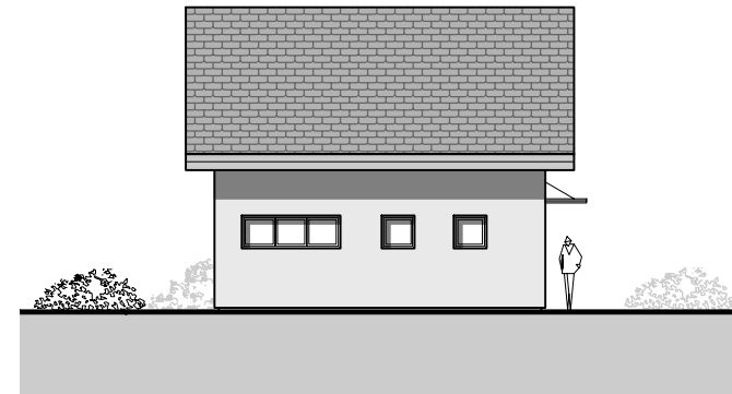
Façade Est
